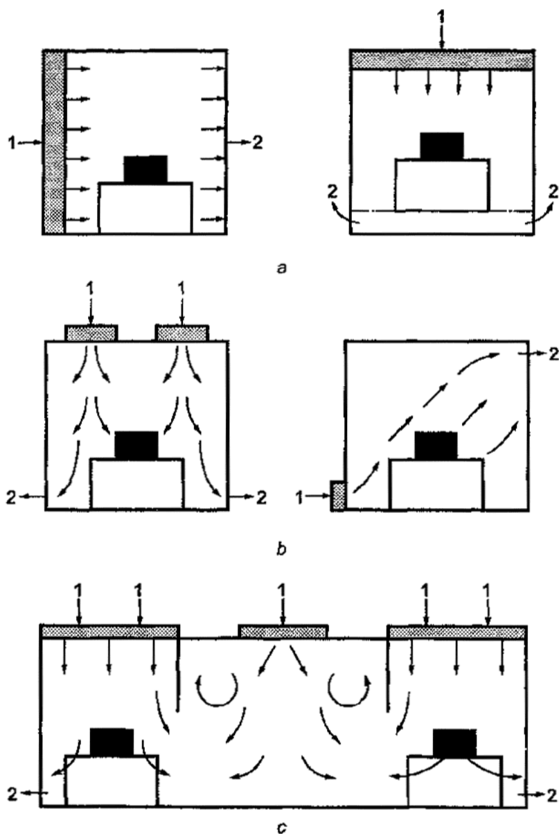
a - односторонний поток воздуха; b - неодносторонний поток воздуха; c - смешанный поток воздуха; 1 - приточный воздух; 2 - вытяжной воздух
